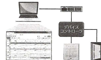
コストを抑えた1扉だけの入退室管理システム「Acsaran-Lite」の構成イメージ図
